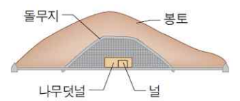
<돌무지덧널무덤 구조>
