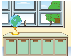
▲ (라)의 위치에서 관측자 모형이 본 교실의 모습
