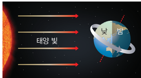
▲ 지구의 낮과 밤
