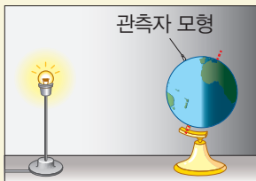
▲ 낮일 때 관측자 모형의 위치
