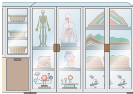
▲ (가)의 위치에서 관측자 모형이 본 교실의 모습
