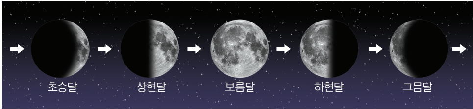
▲ 여러 날 동안 관찰한 달의 모양 변화
